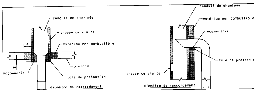
Exemple d'un raccordement au conduit de cheminée
