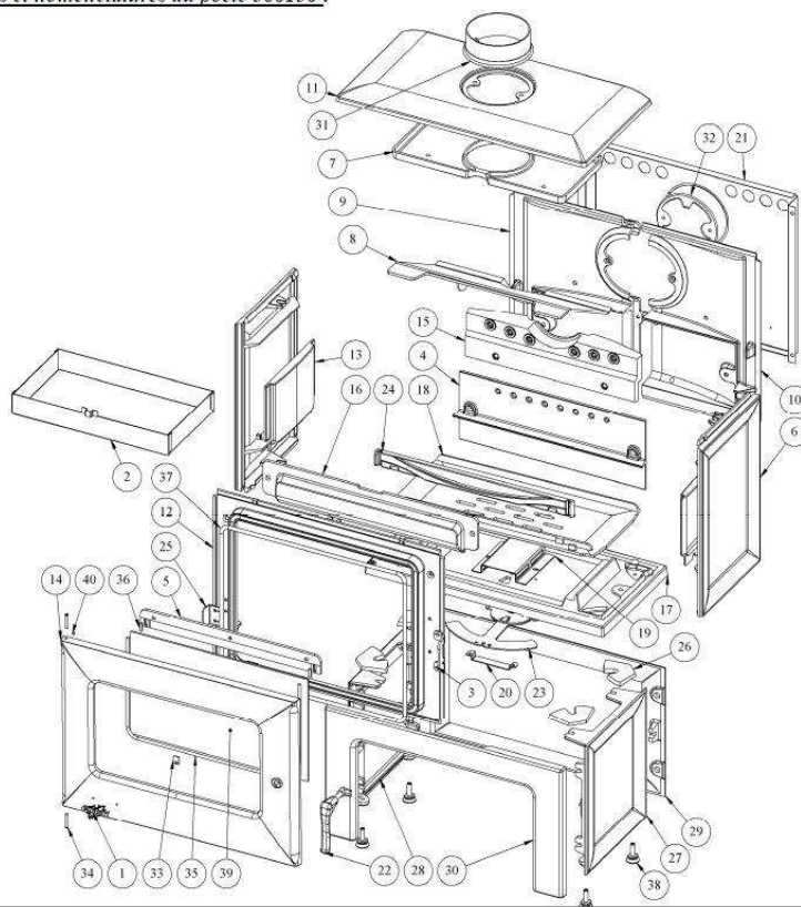
Éclaté et nomenclatures du poêle 388138 :
