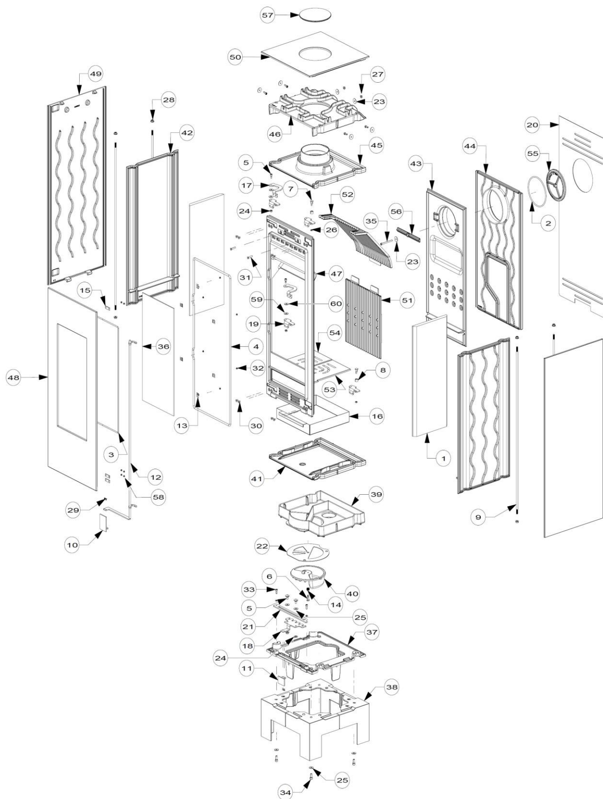
Vue éclatée
