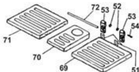
Ensemble couvercle pour 9435.H - 9444.H - 9454.H
