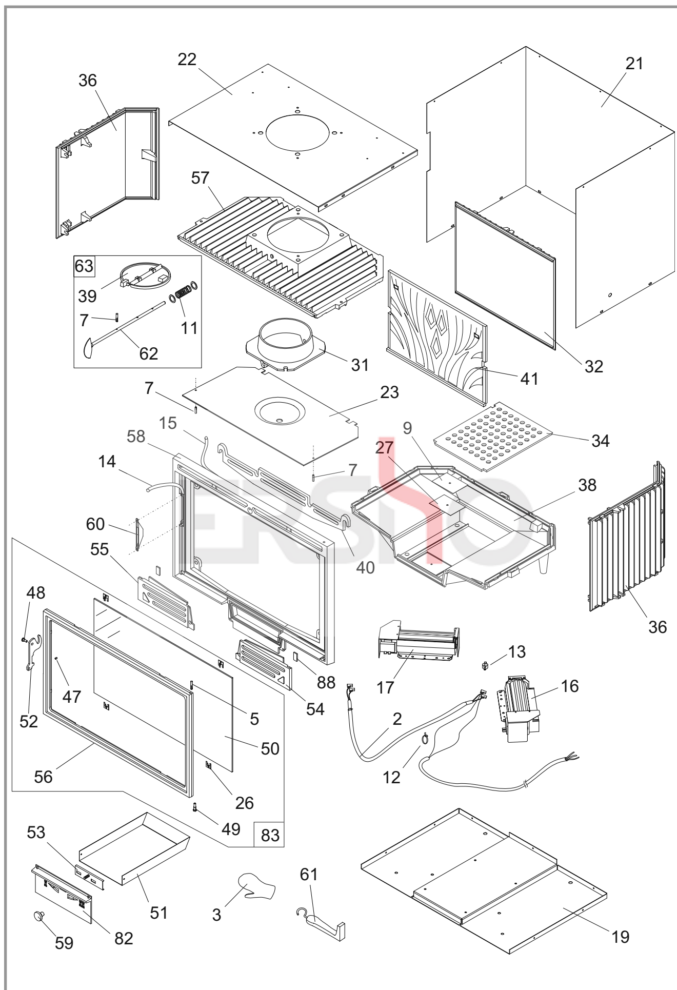
Figure 14 - Vue éclatée de l'appareil 134 10 14 F &amp; C
