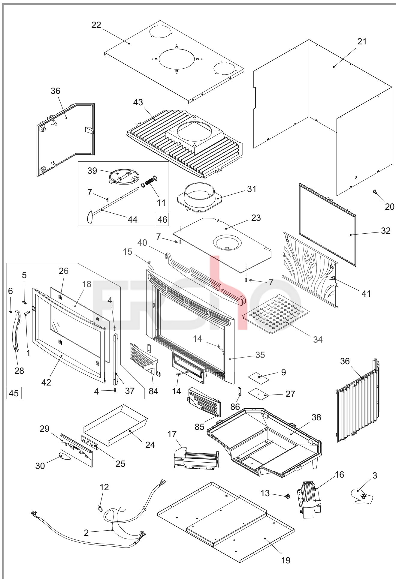
Figure 13 - Vue éclatée de l'appareil 134 10 21 Y
