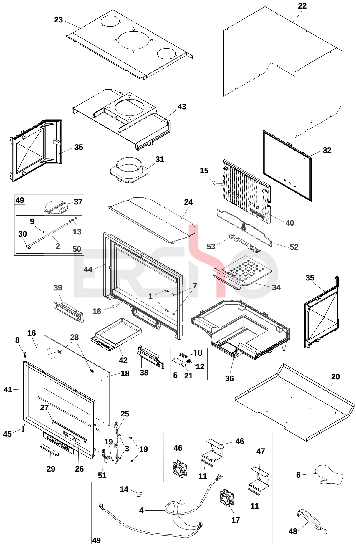
Figure 16 - Vue éclatée de l'appareil
