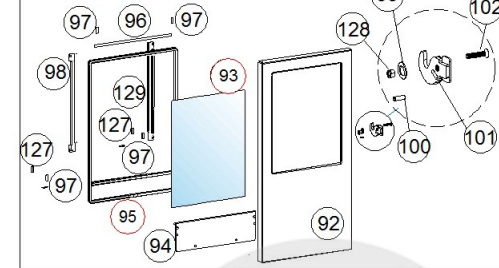
Assieme antina cod. 68069C
