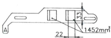
Detail af sekundær og primær luftspjæld
