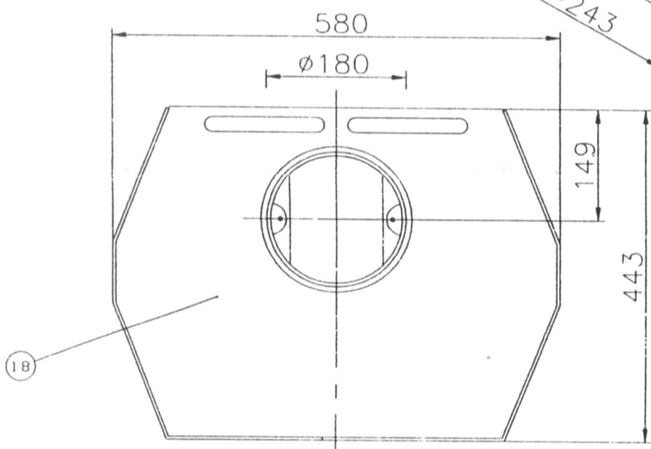
Detail af sekundær og primær luftspjæld
