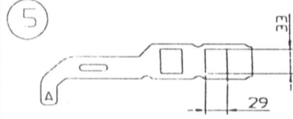
Detail af luftspjæld
