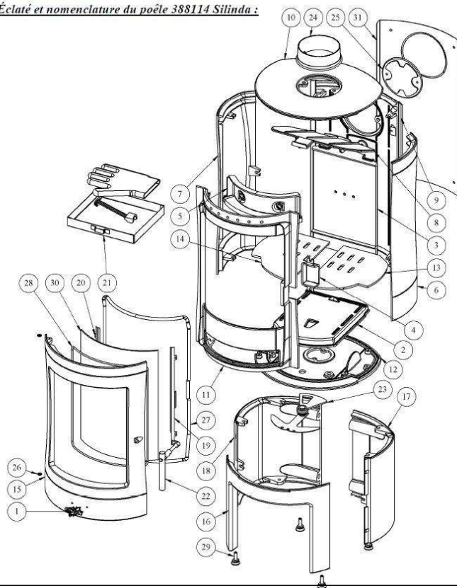
○ Éclaté et nomenclature du poêle 388114 Silinda :
