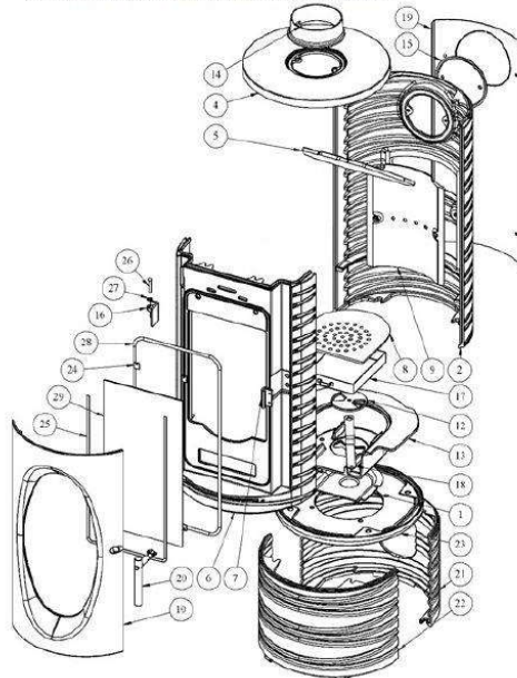
Éclaté et nomenclature du poêle 420012 Talisman :
